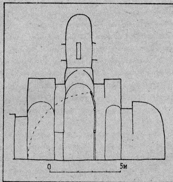
Рис.2. Продольный разрез ц.Никола в Гостинополе. Реконструкция иконостаса.
